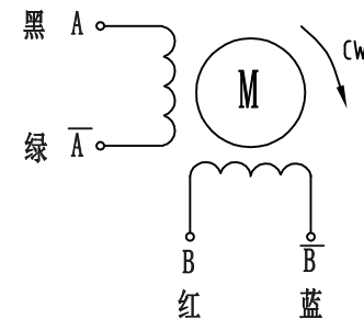
Wiring Diagram:
